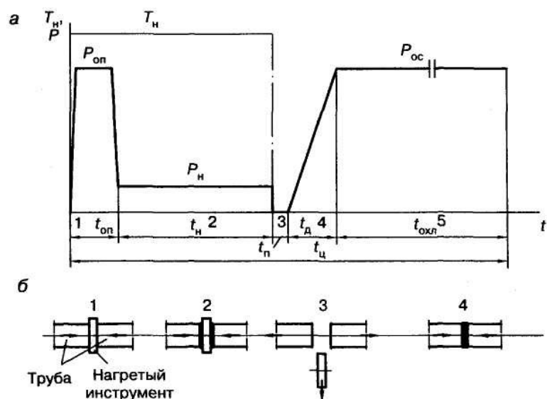
a — диаграмма изменения во времени t давления на торцах P и температуры нагретого инструмента T_n ; б — последовательность протекания процесса сварки; 1 — оплавление торцов; 2 — нагрев концов труб; 3 — вывод нагретого инструмента (технологическая пауза); 4, 5 — осадка и охлаждение стыка
