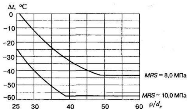
Рисунок 5 —Максимально допустимый отрицательный температурный перепад в зависимости от отношения радиуса упругого изгиба к наружному диаметру газопровода при температуре эксплуатации 0 °С и рабочем давлении 0,6 МПа для SDR 11 и различных MRS
