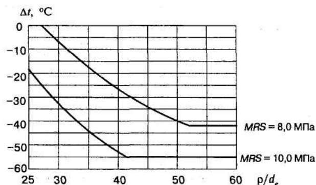
Рисунок 6 —Максимально допустимый отрицательный температурный перепад в зависимости от отношения радиуса упругого изгиба к наружному диаметру газопровода при температуре эксплуатации 0 °С и рабочем давлении 0,3 МПа для SDR 17,6 и различных MRS
