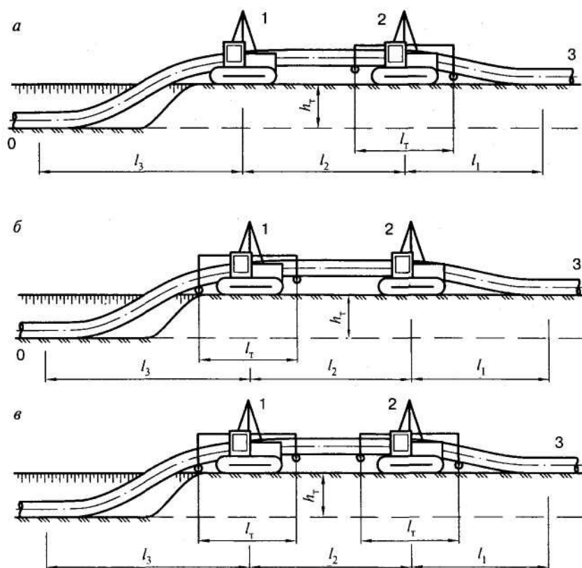
a — с траверсой головного трубоукладчика; б — с траверсой у заднего трубоукладчика; в — с траверсами у обоих трубоукладчиков; 1 — задний трубоукладчик; 2 — головной трубоукладчик; 3 — трубная плеть
